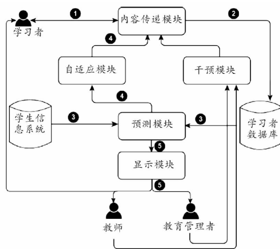
图1 基于大数据的自适应学习系统组成及运行流程
