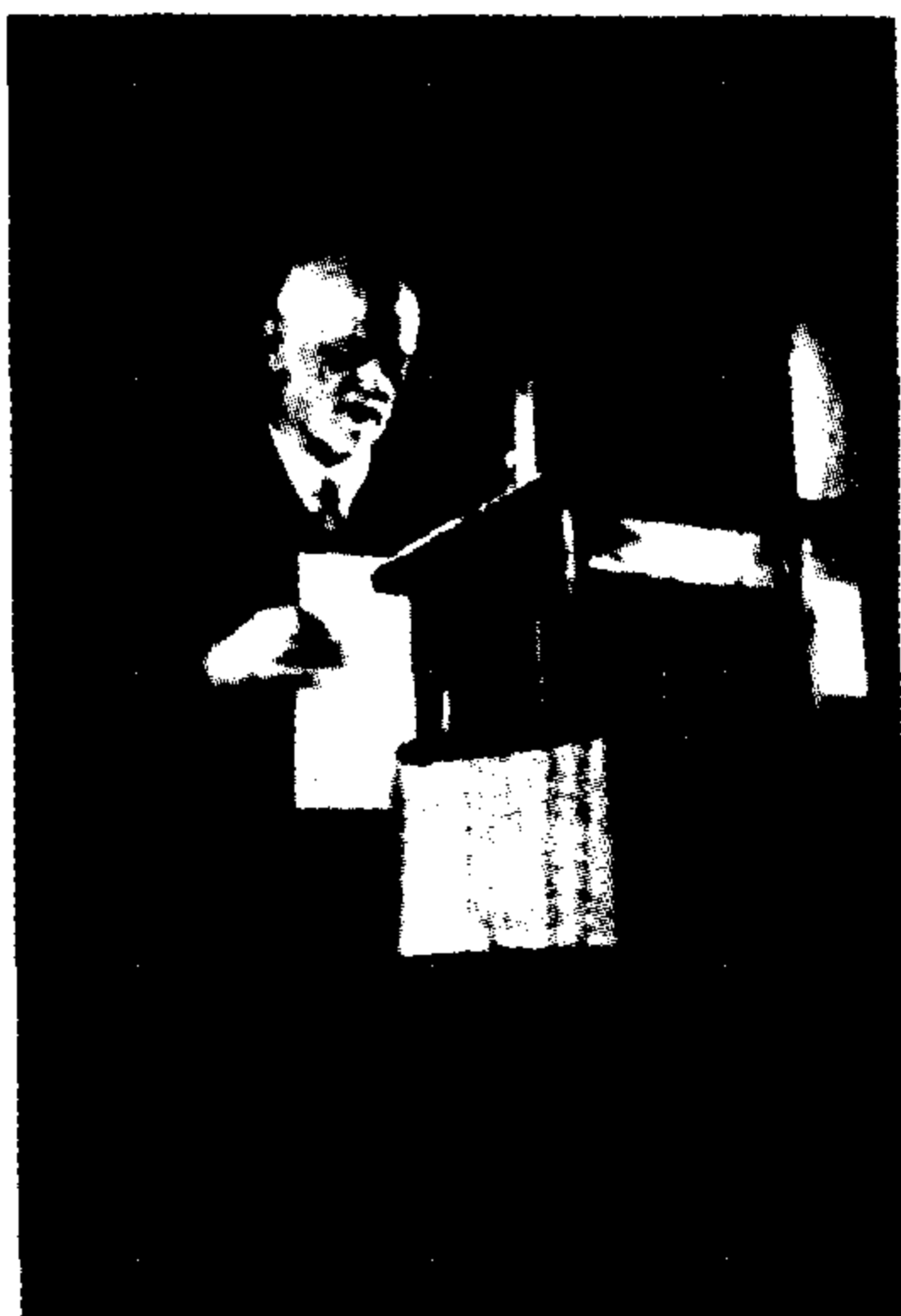
图 11.1 希尔伯特
