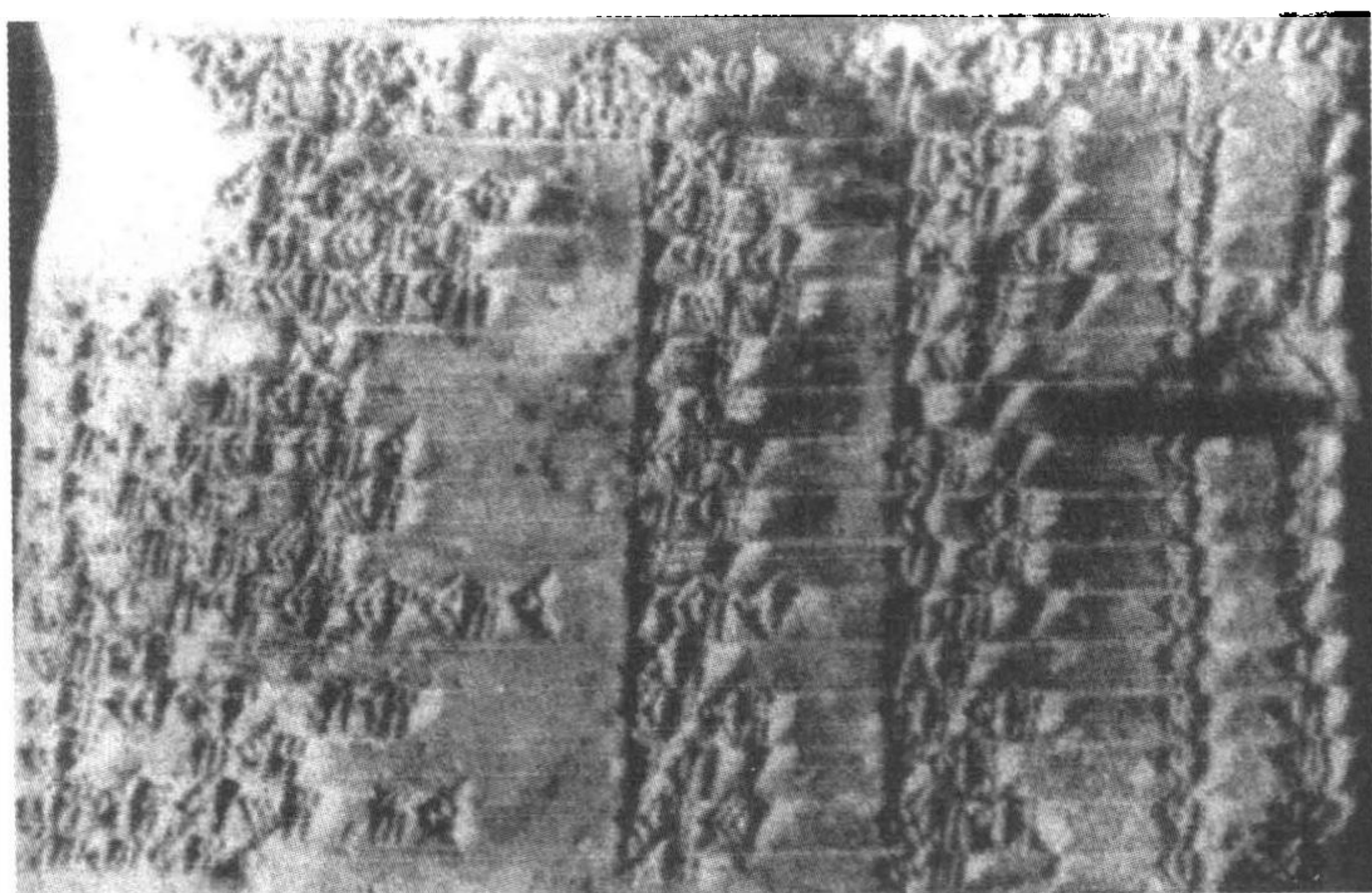
图 1.8 普林顿 322
